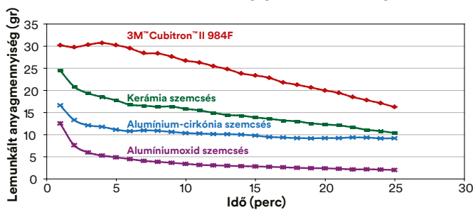
3M™ Cubitron™ II Versenytárs csiszolószalag 1 Versenytárs csiszolószalag 2 Versenytárs csiszolószalag 3 984F 36+
